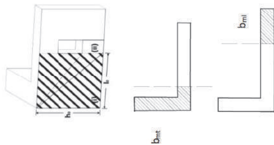
Σχ. Σ 6.11: Ορισμός συνεργαζόμενου μήκους εγκάρσιου προς τον εξεταζόμενο τοίχου.
