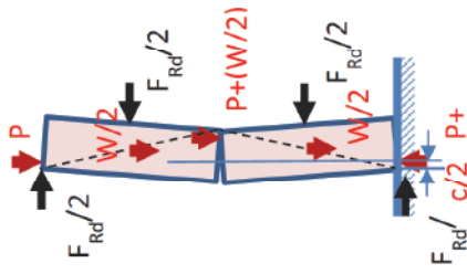
Σχ. Σ 7.8(α): Αντοχή ανατροπής πεσσού, F_R , σε εκτός επιπέδου αστοχία (c το υψος της θλιβόμενης ζώνης).
