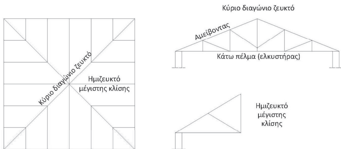
Σχήμα Π.12: Τετρακλινής στέγη επί τετραγωνικής κάτοψης
