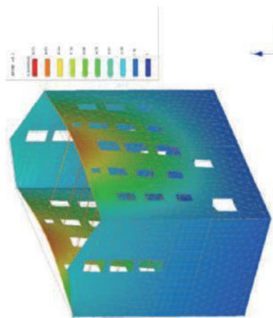
Σχ. Σ 5.11: Μορφολογία προσεγγιστικού σχήματος θεμελιώδους ιδιομορφής που προκύπτει από την επιβολή των βαρυτικών φορτίων στην κατεύθυνση του σεισμού (από το Σχ. Σ 5.10(β)).
