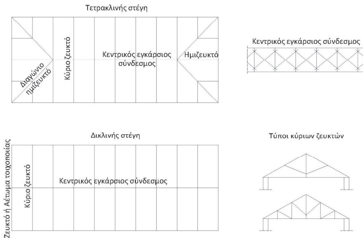
Σχήμα Π.11 : Στέγη επί ορθογωνικής κάτοψης
