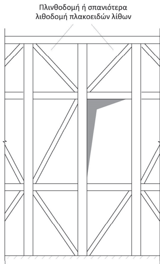
Σχήμα Π.8: Τοιχοδομή με ξύλινο σκελετό και πλήρωση από τοιχοποιία (ξυλόπηκτη ή ξυλόδομητη)
